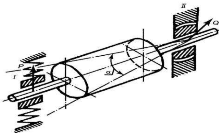
6. Схема колебаний детали при динамической балансировке.
