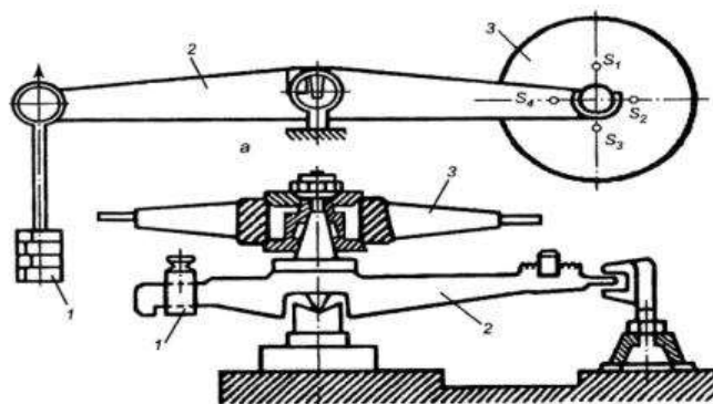
Рис. 5. Схема балансировочных весов для небольших (а) и крупногабаритных (б) деталей: 1 — уравновешивающие грузы; 2 — коромысло; 3 — балансируемая деталь
