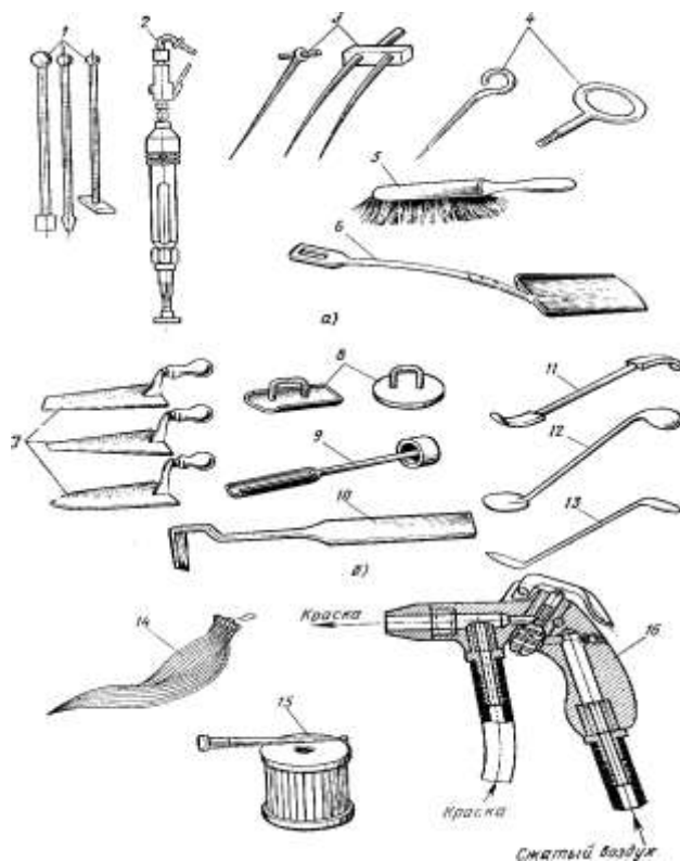
Рис. 2 Инструменты для изготовления (а), отделки (б) и окраски (в) форм: 1- ручные трамбовки, 2- пневматическая трамбовка, 3-душники, 4- винтовые подъёмы, 5- щётка, 6-лопата, 7-плоские гладилки, 8-фасонные гладилки, 9-торцовая гладилка, 10-крючок, 11-полозок, 12-ложечка, 13-ланцет, 14-кисть пенковая, 15-пульверизатор для мелких форм, 16-пульверизатор для крупных форм
