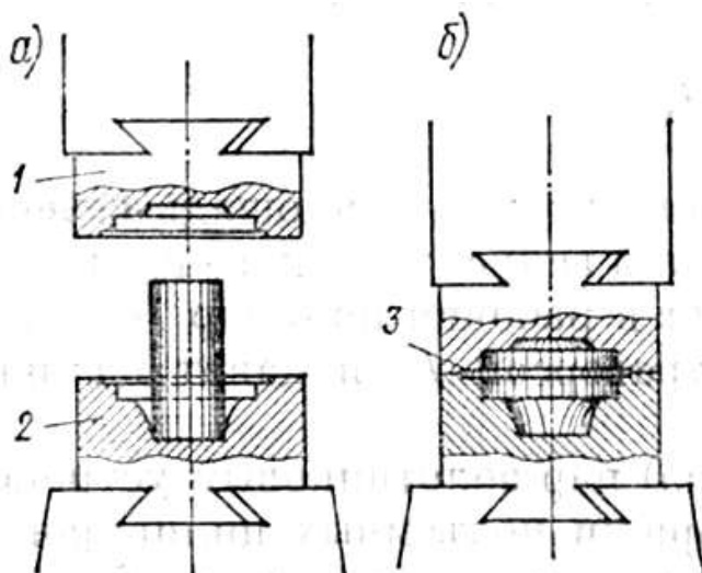
Рис.9 Схема одноручьевого штампа: 1-верхний штамп;2-нижний штамп
