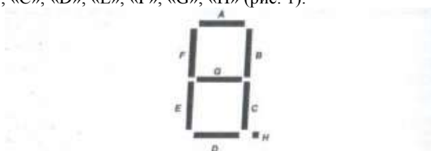
Рис. 1. Внешний вид и структура семисегментного индикатора
