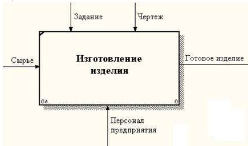
Рис. 3. Контекстная диаграмма
