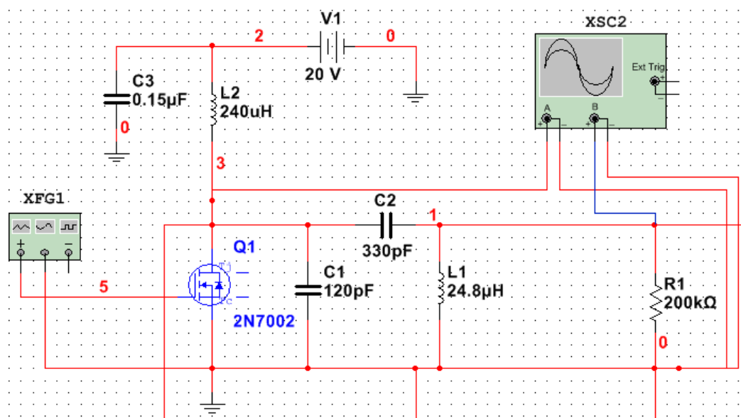
Рис. 1 - Усилительный каскад с LC-цепочкой.
