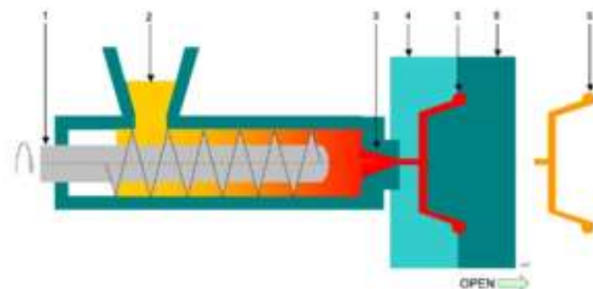
1 — шнек , 2 — дозирующее устройство гранулята, 3 — сопло , 4,6: — две половины пресс-формы, 5 — (красным) полость формы с каналами, 5 — (жёлтым) готовый отлив ок Рисунок 3.1 – Технологическая схема работы термопластавтомата.
