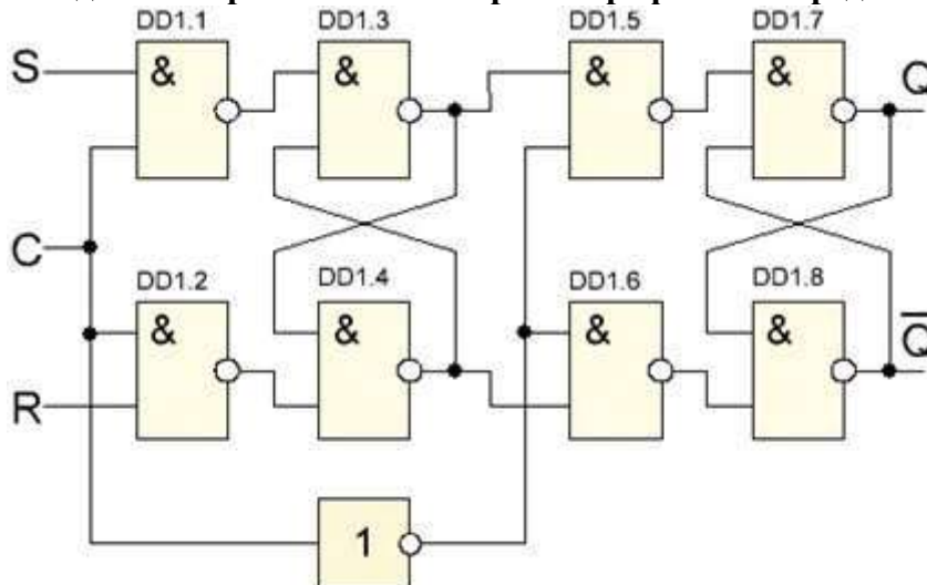
Рисунок 2 – RS-триггер
