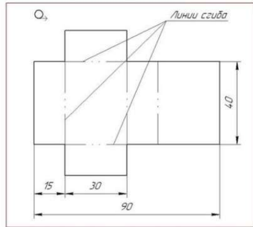
Геометрическое тело №3
