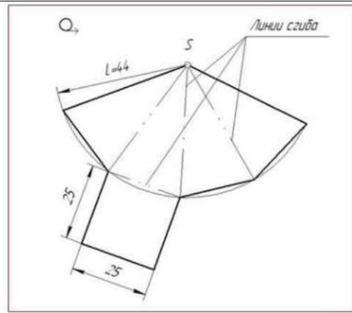
Геометрическое тело №4
