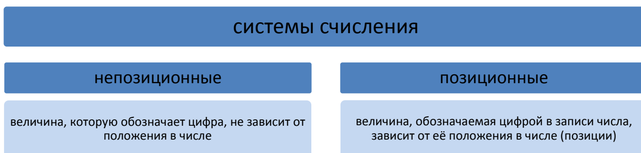
Рисунок 4 – Системы счисления
