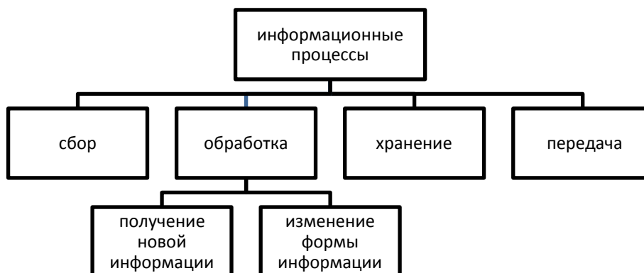
Рисунок 5 – Информационные процессы
