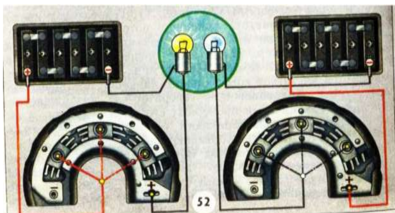
Рисунок 26. Проверка диодов плюсовой шины выпрямительного блока типа ВВГ прямым (слева) и обратным (справа) включением шины в цепь
