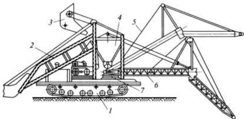
Рисунок 3. Самоходный бетоноукладчик.
