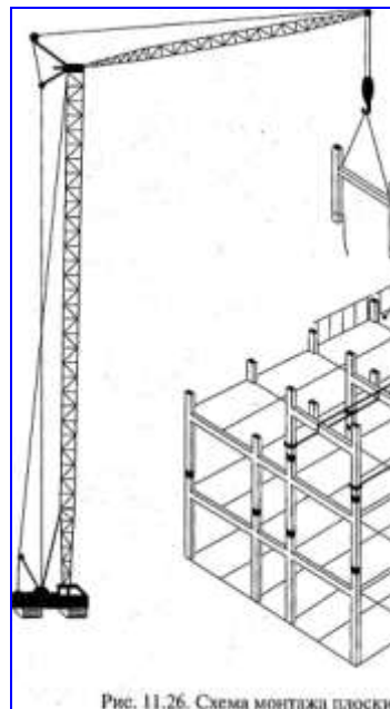
Рис. 11.26. Схема монтажа плоских Н – образных рам.
