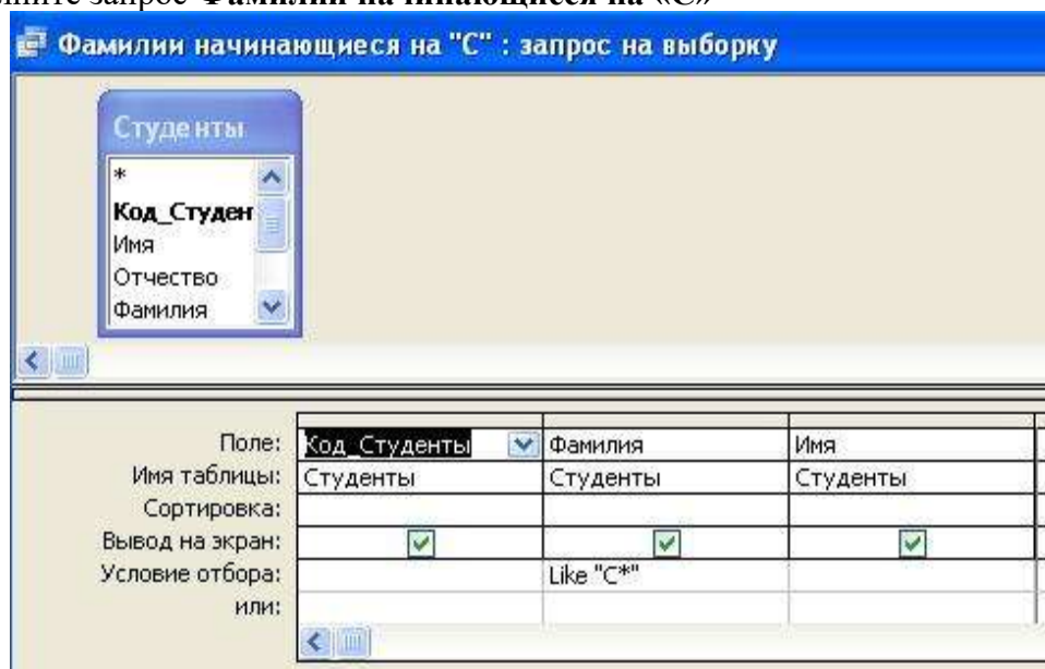
Рис. 1. Форма запроса студентов, фамилии которых начинаются на букву «С»
