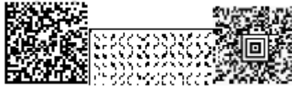
Рисунок 2 – Двухмерный штрих-код
