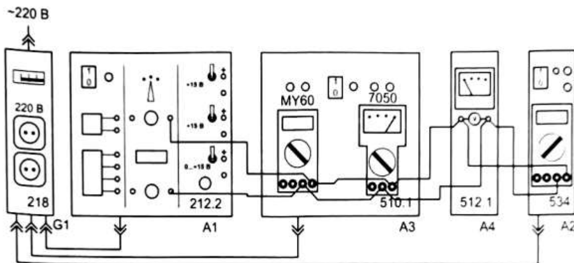
Рис. 2 – Схема электрическая соединений для измерения несинусоидального напряжения
