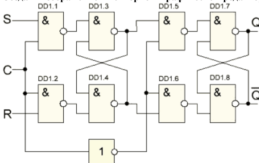
Рисунок 2 – RS-триггер
