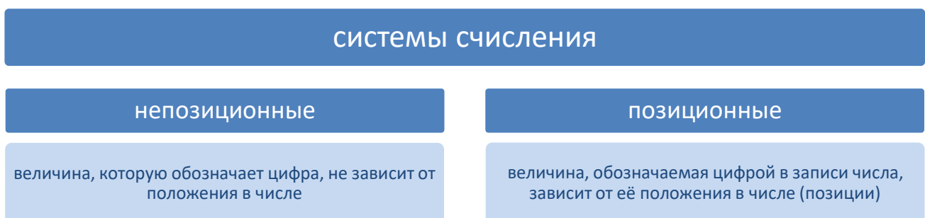
Рисунок 4 – Системы счисления
