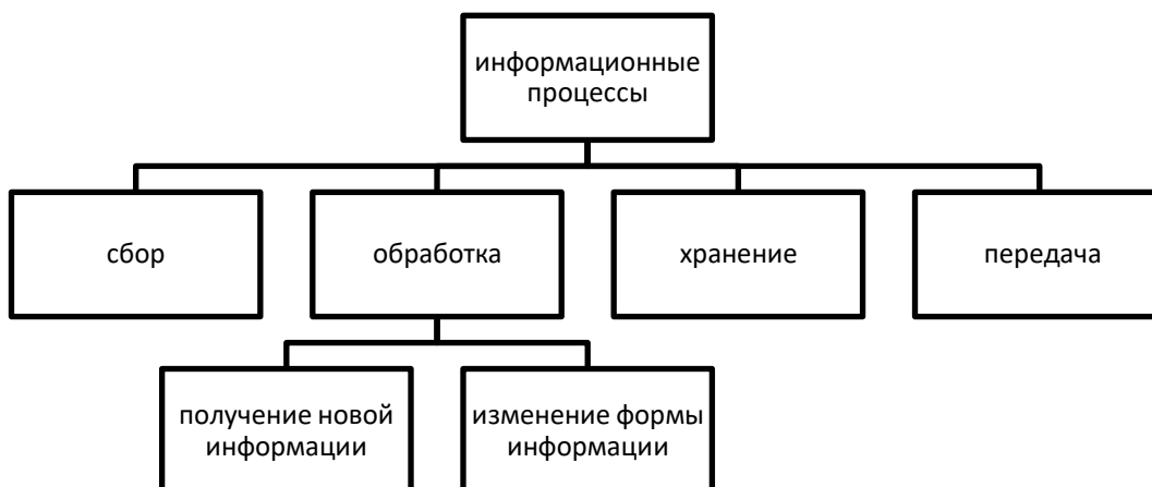
Рисунок 5 – Информационные процессы
