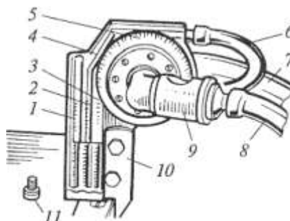
Рисунок 1-Прибор КИ-4887-1 для определения технического состояния цилиндропоршневой группы двигателей:
