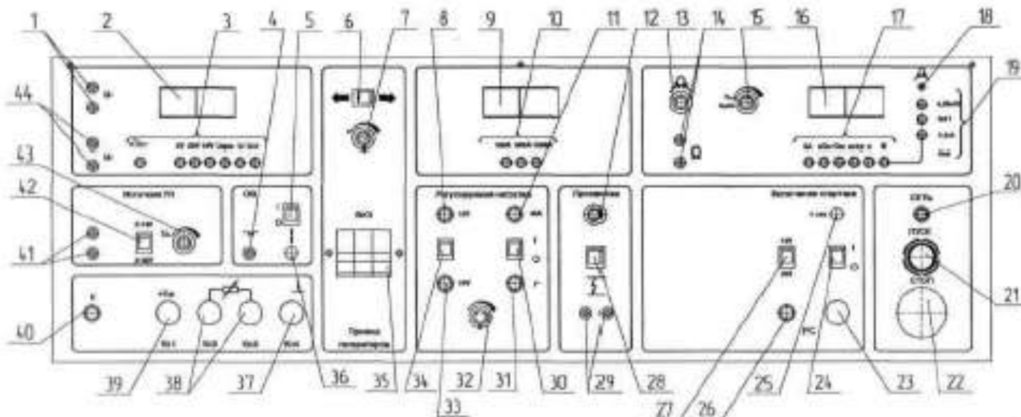
Рисунок 5. Панель управления:
