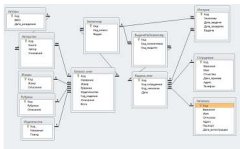
Рисунок 5 – Схема алгоритма
