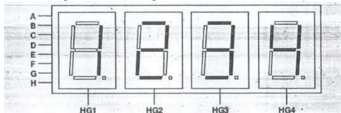
Рис. 5. Схема реализации динамической индикации символов
