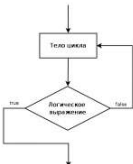
Цикл repeat
