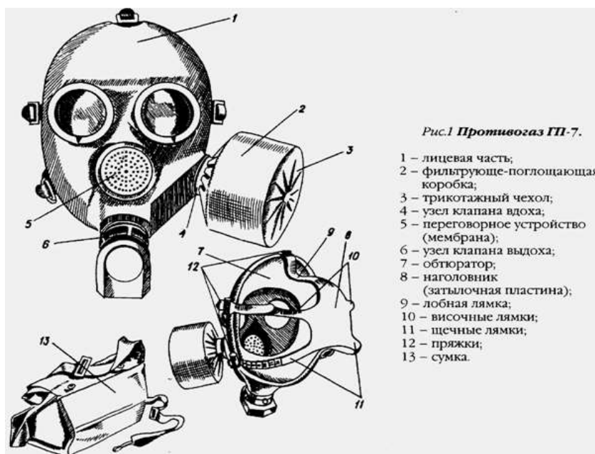
Рисунок 1 Противогаз ГП-7.
