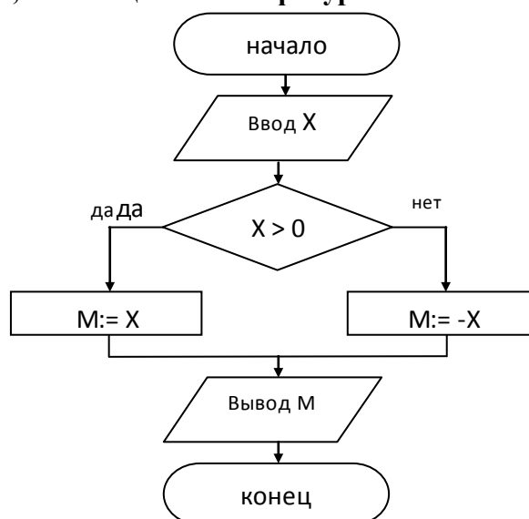
Рисунок 1 – Разветвляющийся алгоритм
