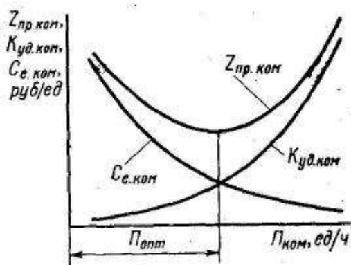
Рис. 4 Функциональная зависимость производительности комплекта P_{ком} машин от себестоимости единицы его продукции C_{с.ком} , удельных капиталовложений K_{уд.ком} и приведенных затрат Z_{пр.ком}
