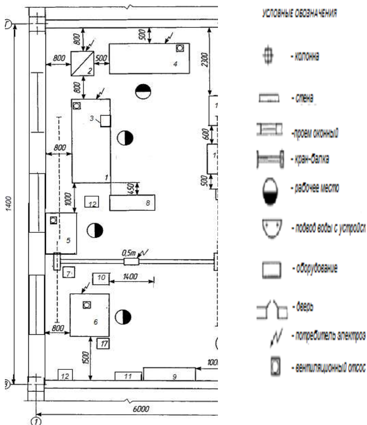
1 - Токарно-винторезный станок 16К20
