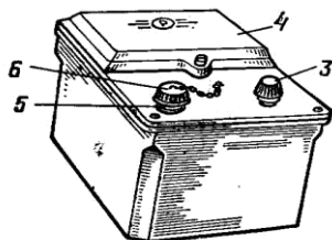
1 – зарядное устройство ЗД-5; 2 – индивидуальные дозиметры ДКП-50-А; 3 – ручка потенциометра; 4 – крышка отсека питания; 5 – зарядное гнездо; 6 – колпачок Рис. 2 – Комплект индивидуальных дозиметров ДП-22В
