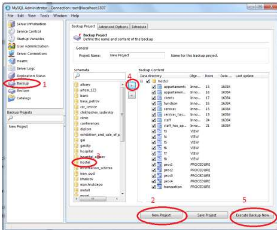
Рисунок 2 - Шаги выполнения резервной копии
