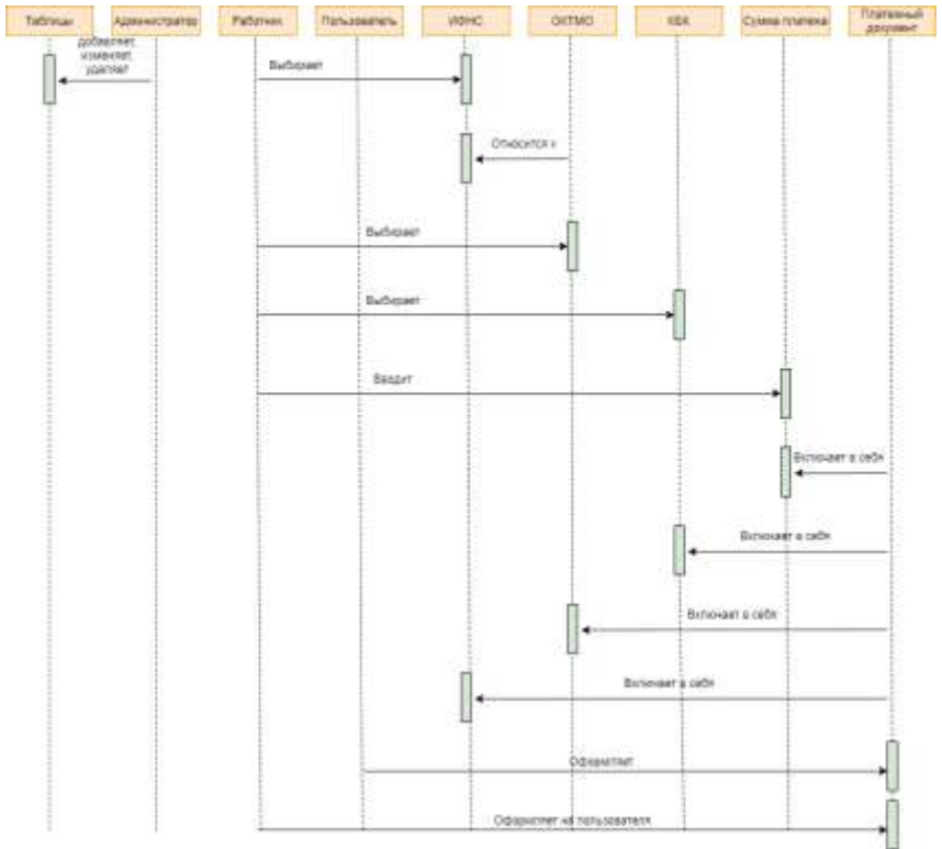
Рис. 4.3. Диаграмма последовательностей
