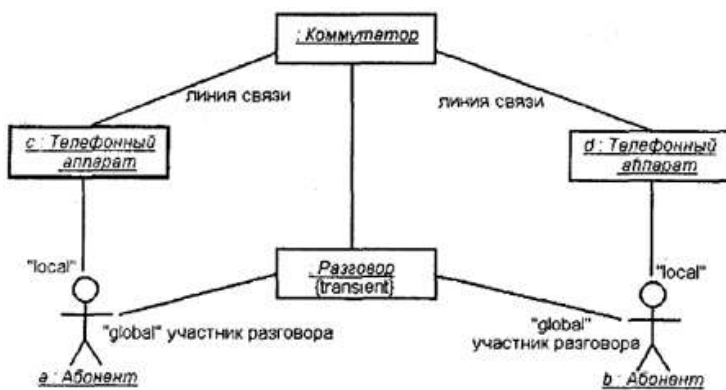
Рис. 9. фрагмент диаграммы кооперации, дополненный стереотипами ролей связей, именами ассоциаций и помеченным значением объекта.
