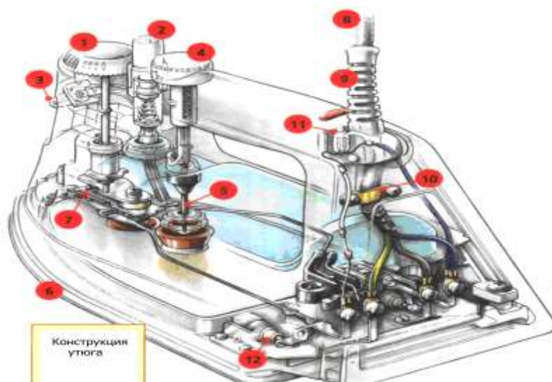
Рис.2 Конструкция утюга
