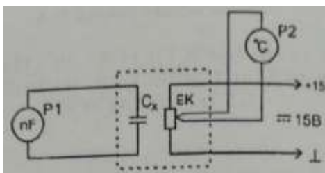
Рис. 2. Схема электрическая соединений типового комплекта для измерения зависимости диэлектрической проницаемости и угла диэлектрических потерь от температуры
