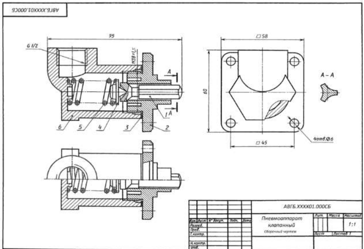
Рис. 10.1 Пневмоаппарат клапанный
