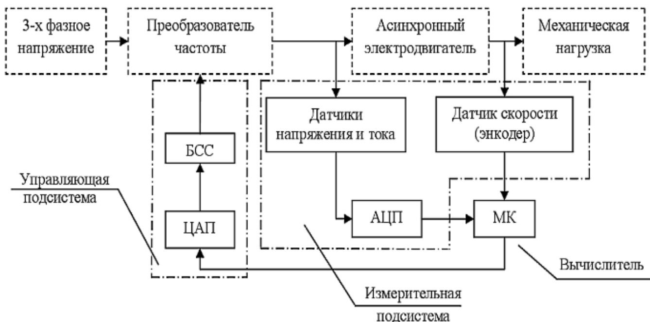
Рисунок 5 – Блок-схема системы стабилизации активной мощности
