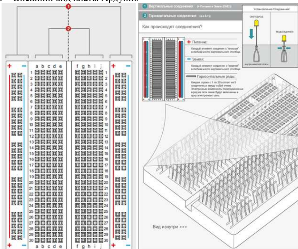
Рисунок 2 – Макетная плата
