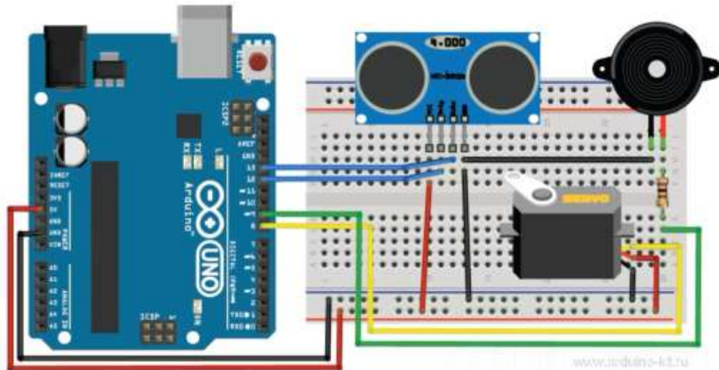
Рисунок 13– Схема сборки
