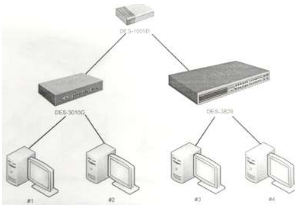
Рисунок 4 -Топология сети
