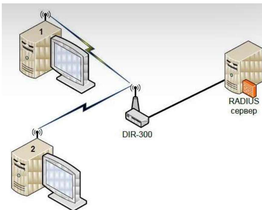
Рисунок 28 – Топология сети
