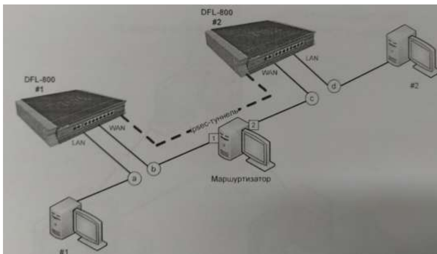
Рисунок 39 – Топология сети
