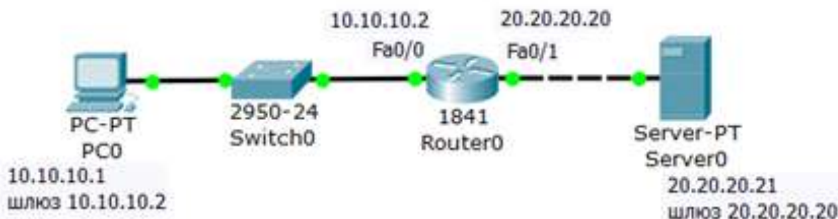
Рисунок 30 - Схема сети
