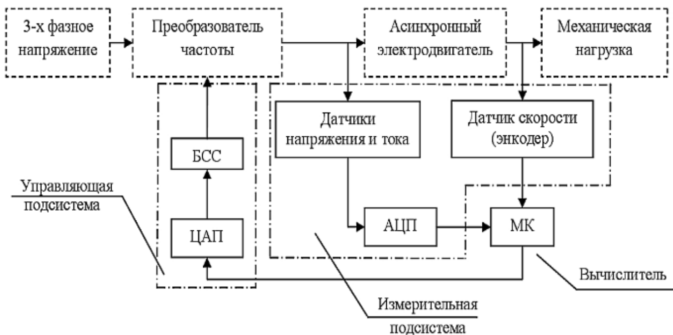
Рисунок 5 – Блок-схема системы стабилизации активной мощности
