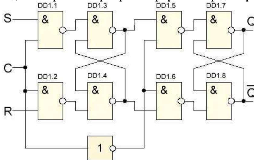
Рисунок 2 – RS-триггер
