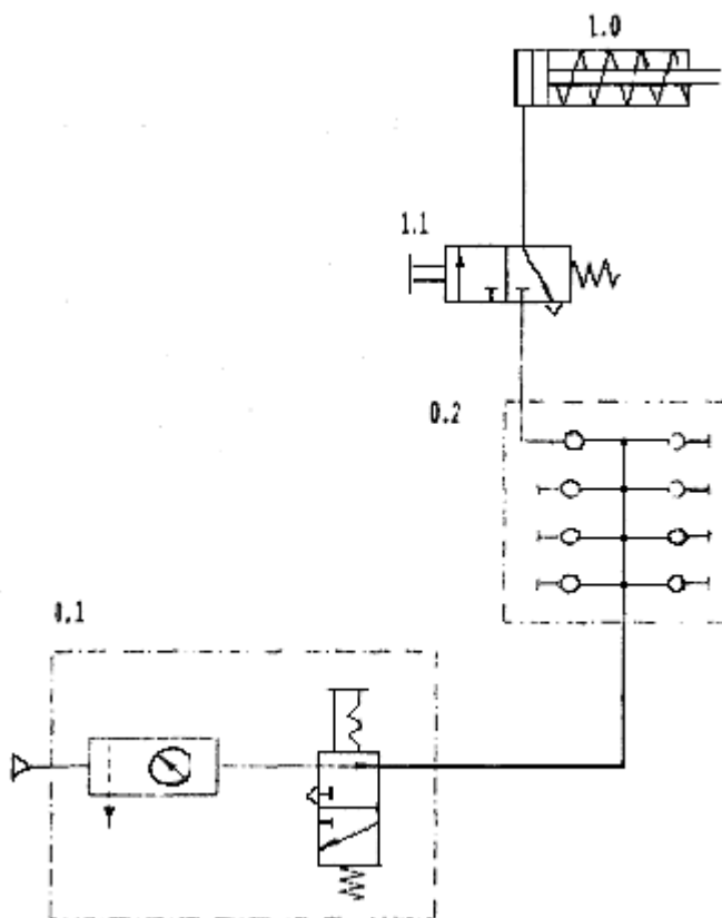
Рисунок 1 - Принципиальная схема
