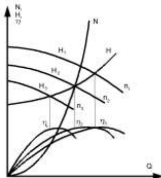
Рисунок 5 – Регулирование изменением числа оборотов насоса.
