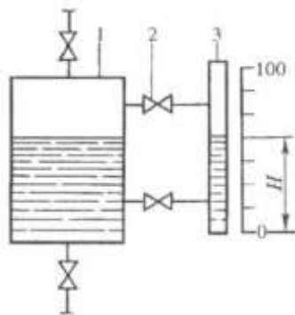
Рис. 1. Визуальный уровнемер.
