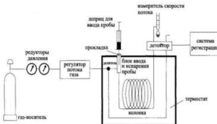
Рис. 2 - Принципиальная схема газового хроматографа: 1 – баллон с газом–носителем; 2 – регулятор расхода; 3 – место ввода пробы (кран–дозатор, испаритель); 4 – термостаты; 5 – колонка; 6 – детектор; 7 – регистратор.
