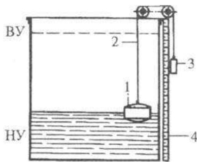
Рисунок 2 - Поплавковые уровнемеры с плавающим поплавком
