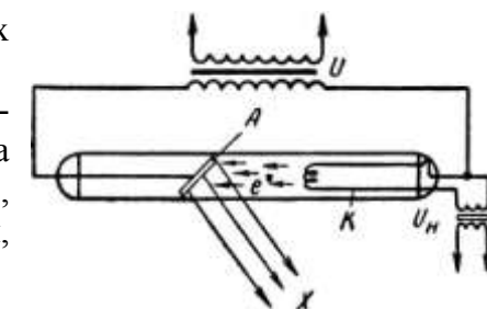
Рис. 2.2. Схема рентгеновской трубки U_n – напряжение накала
