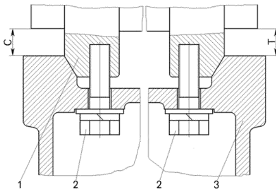
Рис.9.2 - Крепление гидроцилиндра:
