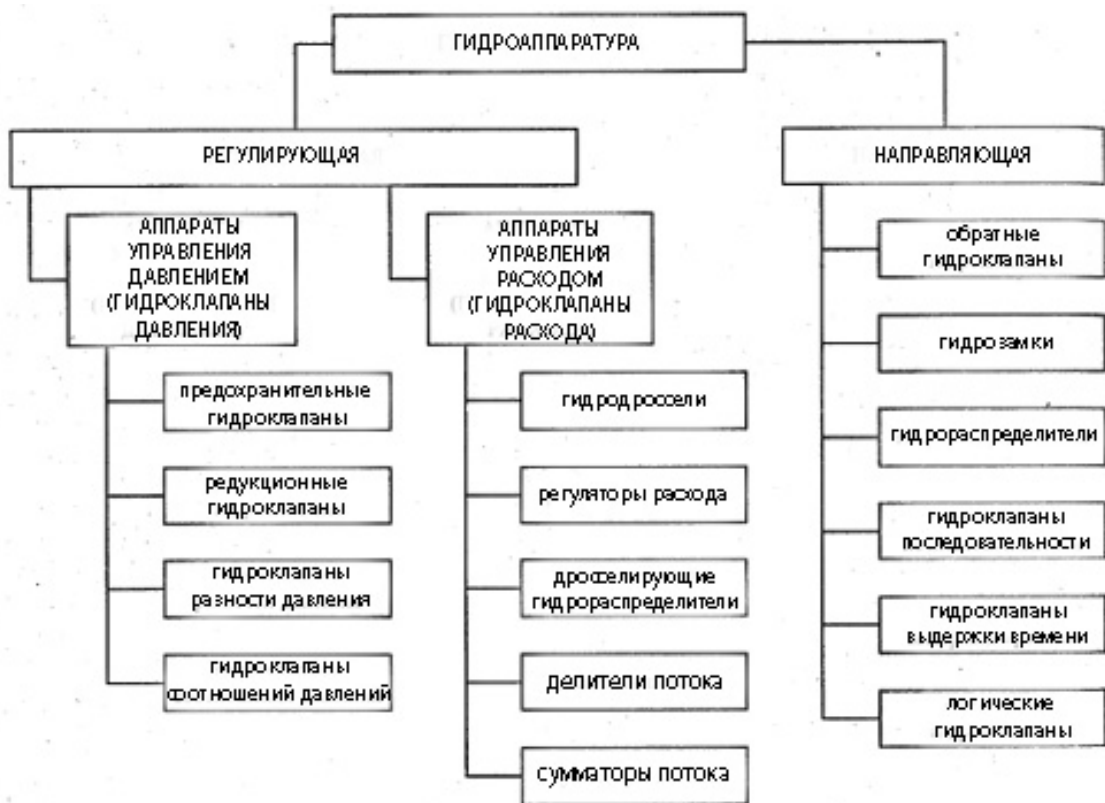
Рисунок 2 – Гидроаппаратура
