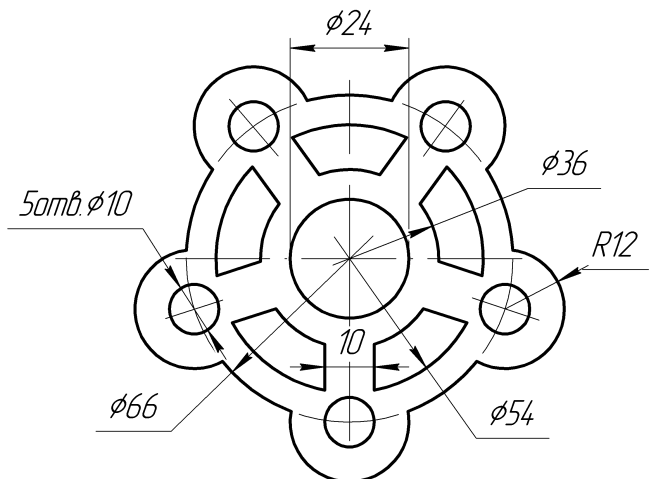
Прокладка
