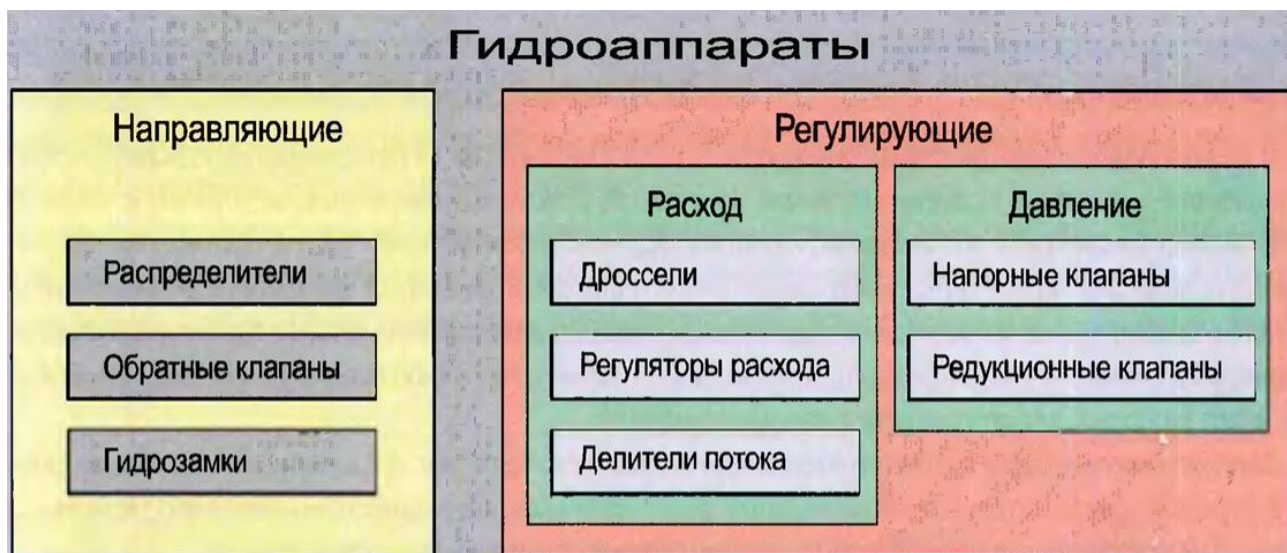
Рисунок 4 – Гидроаппаратура
