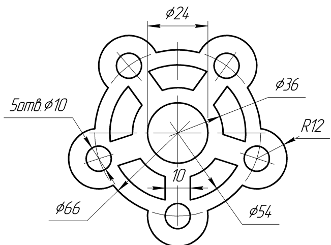
Прокладка
