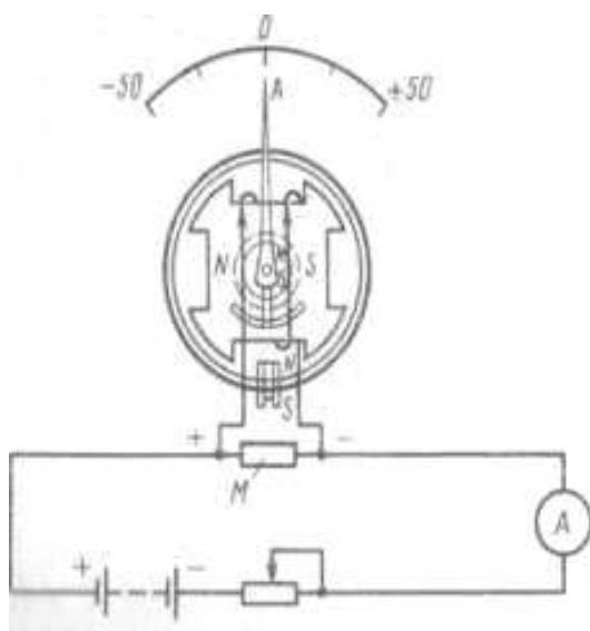
Рис.105 Проверка амперметра
