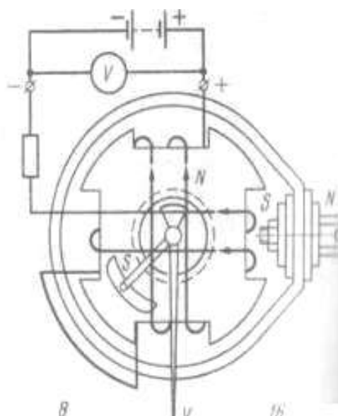
Рис.106 Проверка вольтметра
