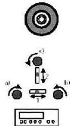
Рис 11. Горизонтирование и точное центрирование
