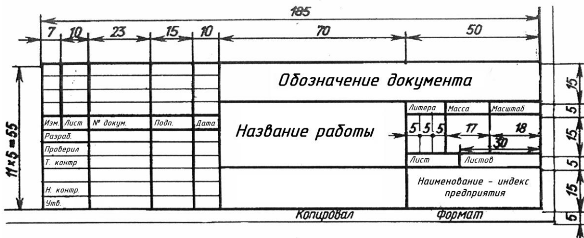
Рисунок 3 - Основная надпись
