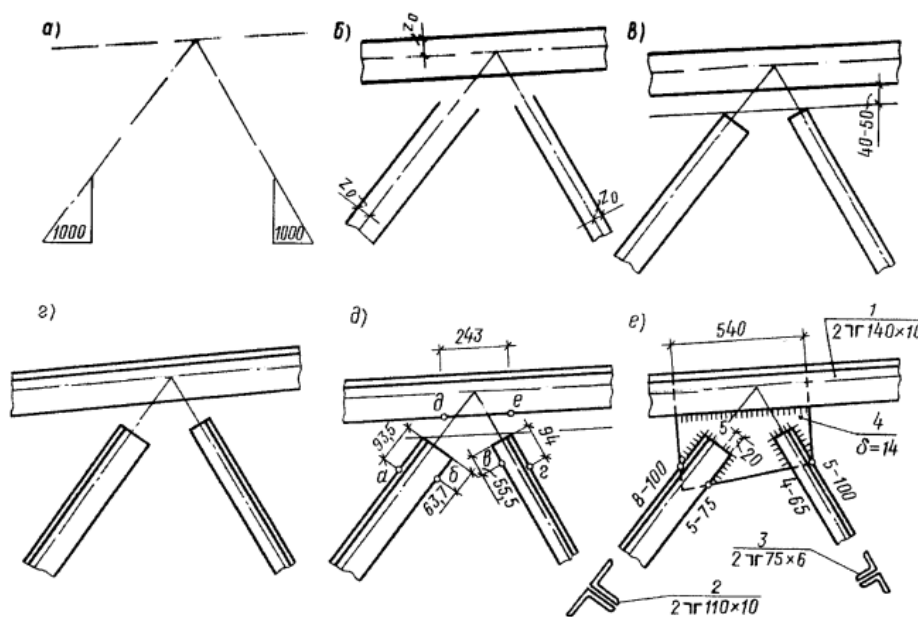
Рисунок 77 - Последовательность построения узла фермы
