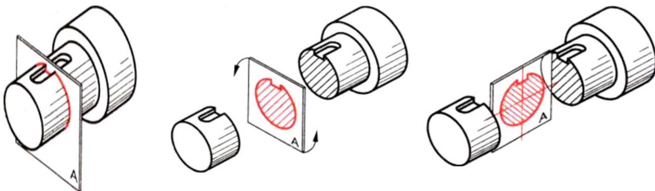
Рисунок 27 - Сечение
