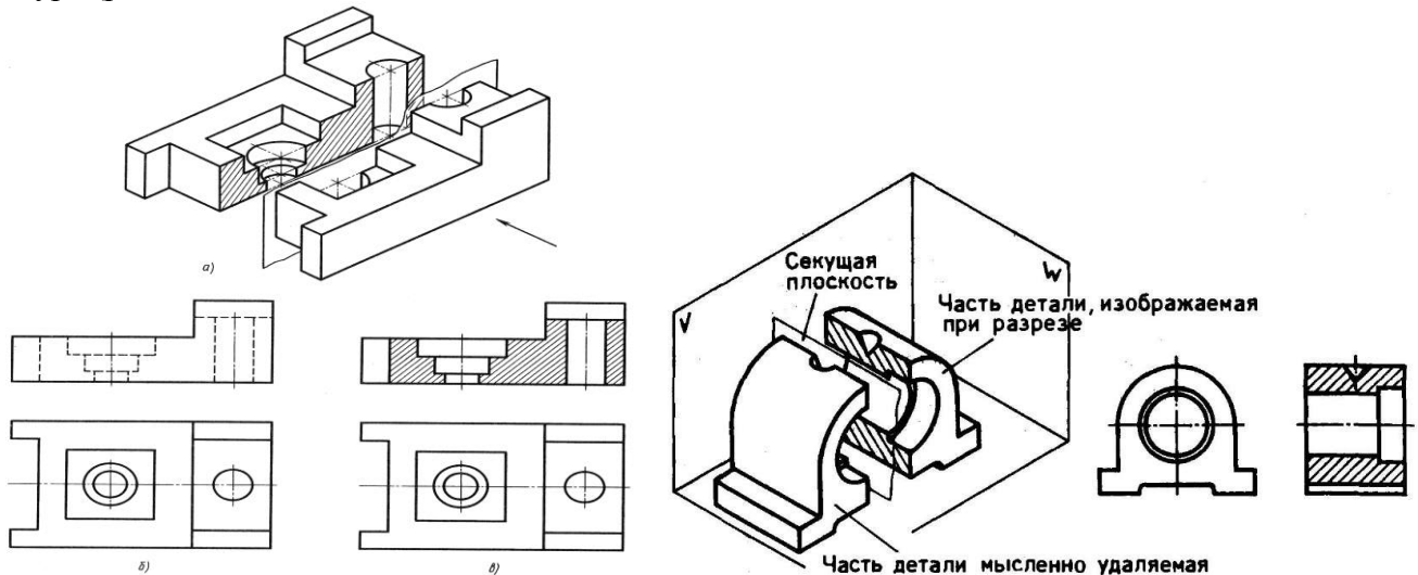
Рисунок 30 - Разрез
