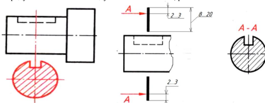
Рисунок 28 – Сечение на продолжении секущей плоскости
