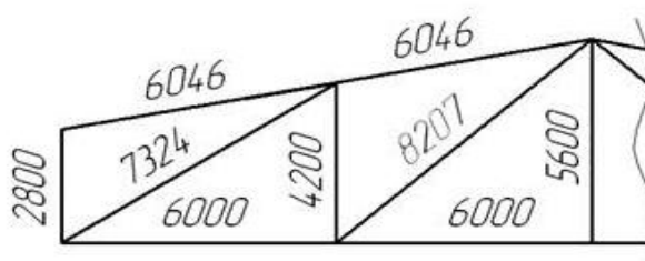
Рисунок 73 - Пример изображения геометрической схемы фермы
