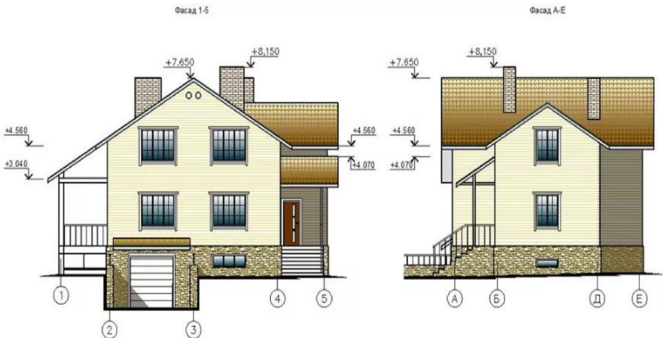
Рисунок 60 - Фасад здания
