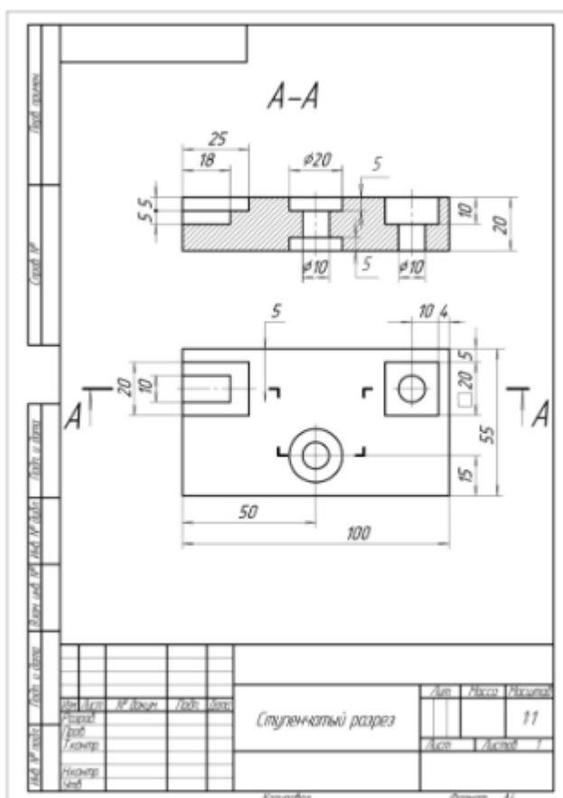
Рисунок 37 – Ступенчатый разрез
