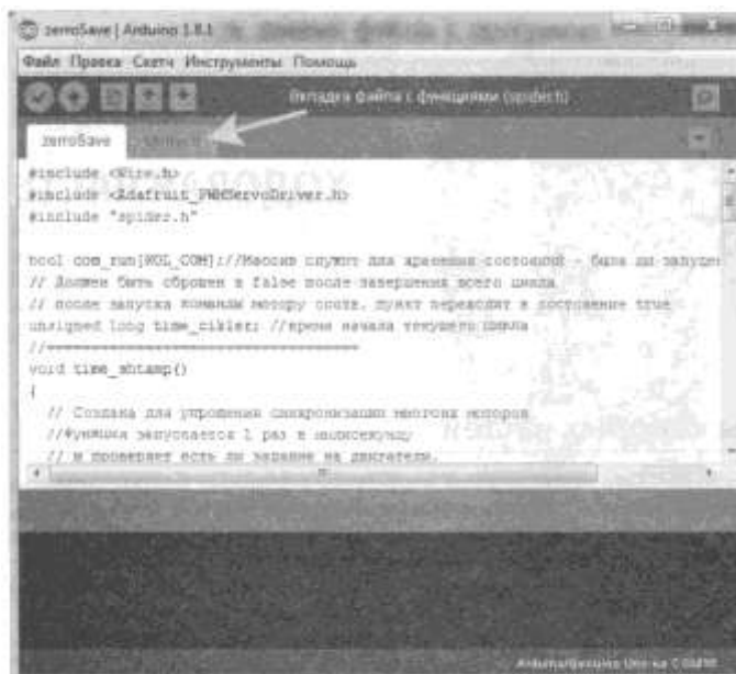
Рис. 4.18. Пример разделения программы на два файла: основной — zeroSave.ino и дополнительный — spidev.h
