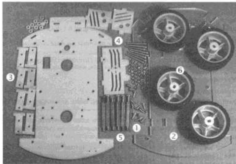
Рис. 6.2. Набор конструкционных деталей: винты и гайки (1); верх корпуса и низ (2); Т-образные элементы для установки двигателей в корпус (3); элементы для установки вращающейся «головы» с датчиком расстояния (4); стойки (5); колеса (6)
