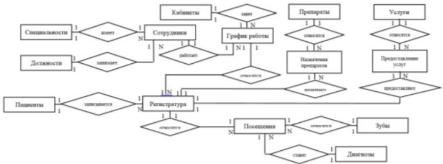
Рис. 4.1. Концептуальная модель
