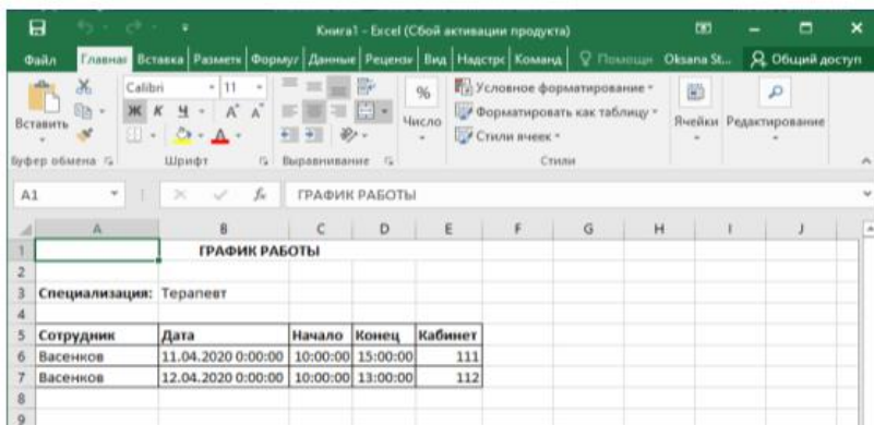
Рис.4.12. Фрагмент отчета
