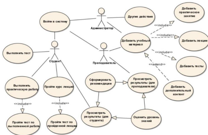
Рис. 4.3 Диаграмма прецедентов
