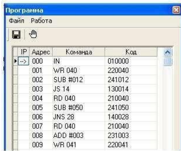
Рис. 10. Окно Программа
