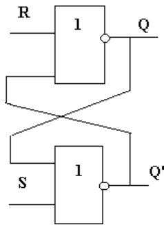
Рис. Асинхронный R-S триггер на логических элементах "ИЛИ-НЕ"
