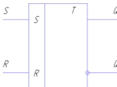
Синхронный R-S -триггер с прямыми входами.
