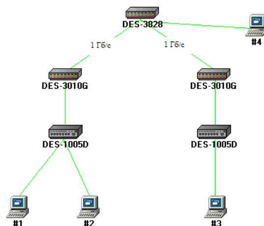
Рисунок 1 - Топология коммутуруемой сети
