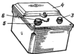
Рис. 2 – Дозиметр карманный прямопоказывающий ДКП-5А
