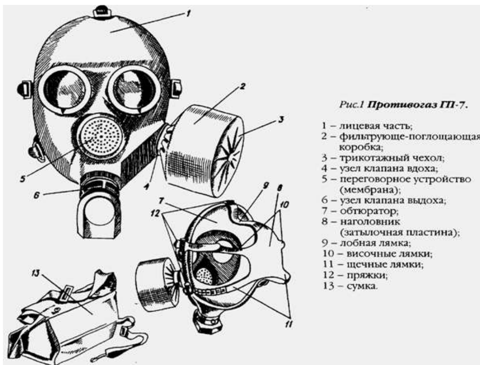
Рисунок 2- Противогаз ГП-7
